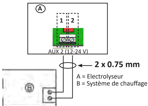
Raccordement d'un système de chauffage avec commande marche/ arrêt à distance
