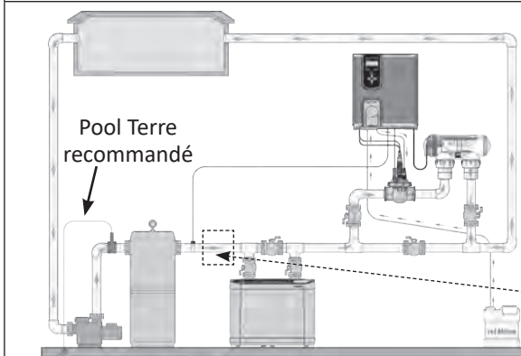
Installation avec un système de chauffage
