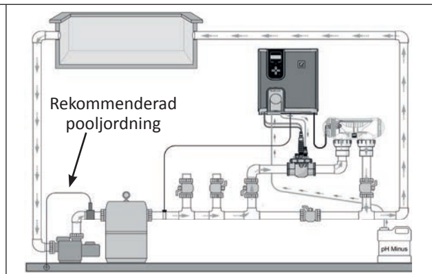
Installation över bypass
